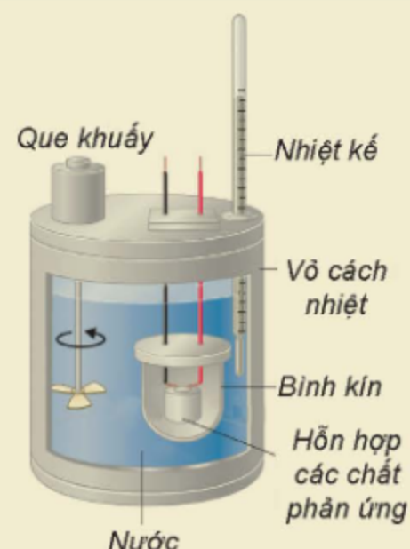
Hình 17.2. Một mô hình nhiệt lượng kế
