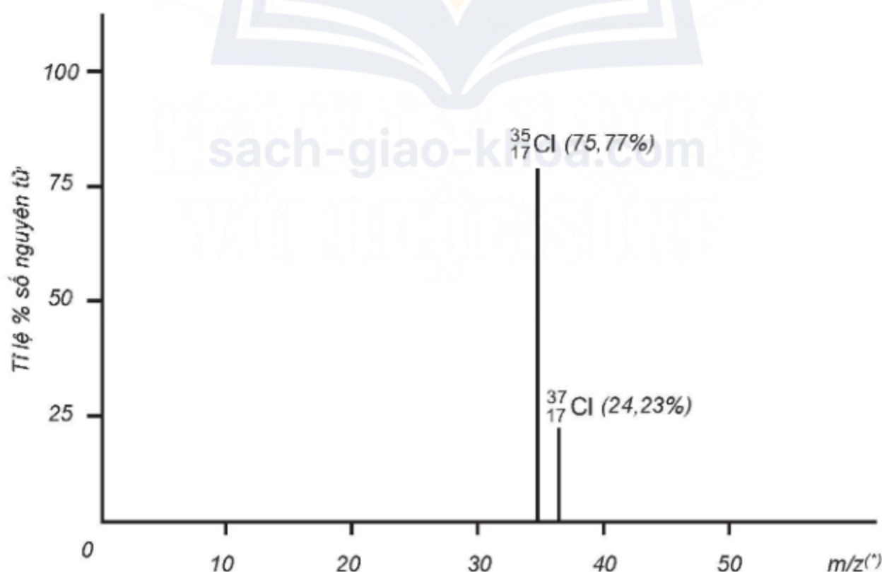
Hình 2.3. Phổ khối lượng của chlorine
