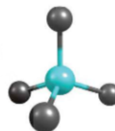
Mô hình phân tử AX_4
