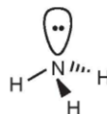
Sơ đồ phân tử NH_3
