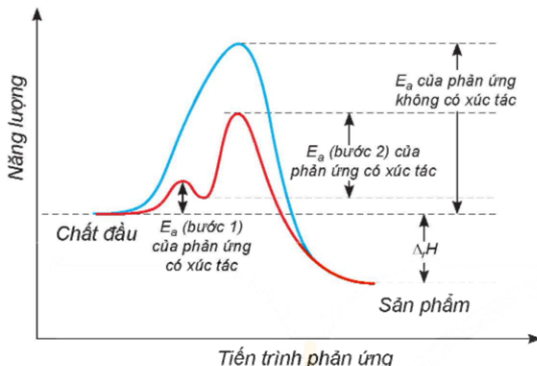
Hình 3.1. Ảnh hưởng của xúc tác đến năng lượng hoạt hoá
