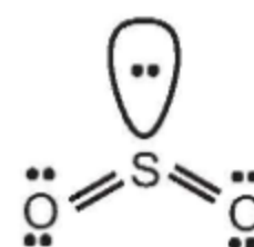
Sơ đồ phân tử SO_2
