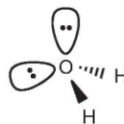
Sơ đồ phân tử H_2O
