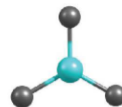
Mô hình phân tử AX_3
