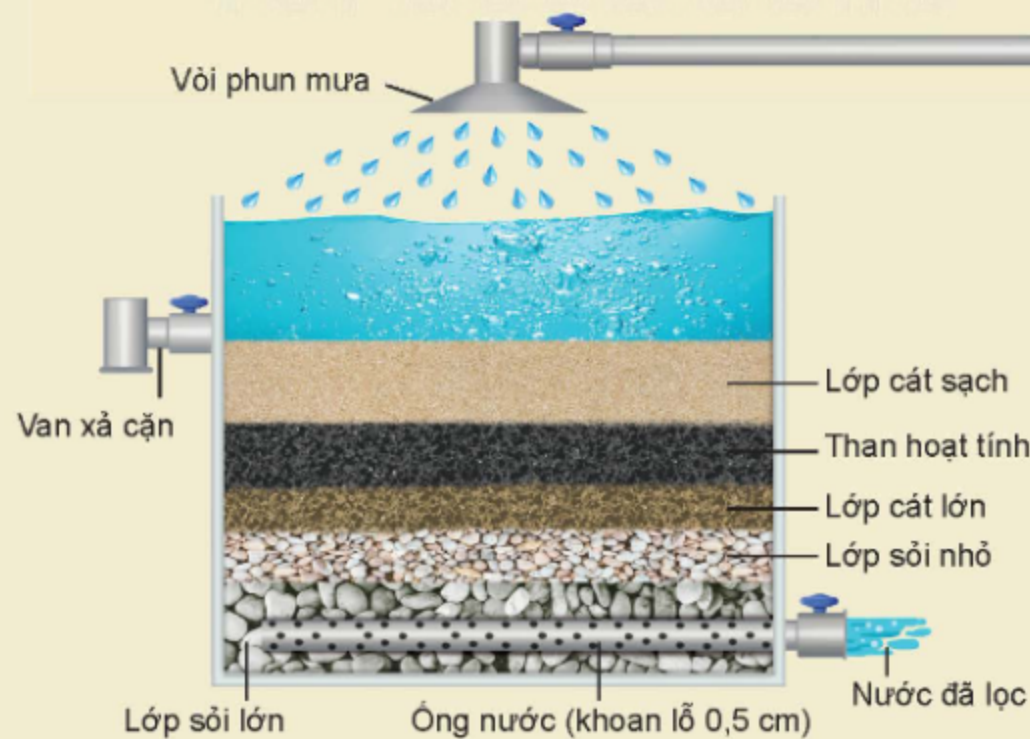
Hình 6.4. Cấu tạo bể lọc nước gia đình
