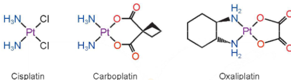
Hình 9.2. Ba phức chất của Pt^{2+} được dùng làm thuốc chữa bệnh ung thư (1)
