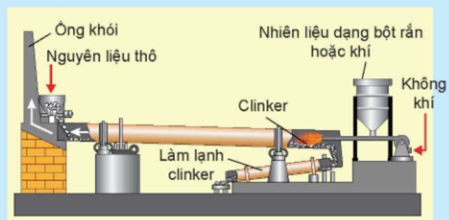
Hình 5.6. Sơ đồ dây chuyền sản xuất clinker
