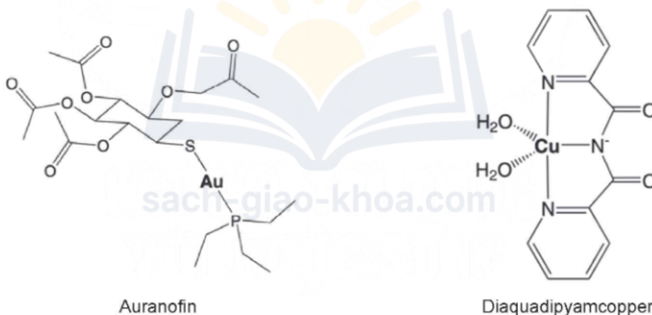
Hình 9.3. Phức chất của Au^+ được dùng làm thuốc chữa bệnh thấp khớp (2)
