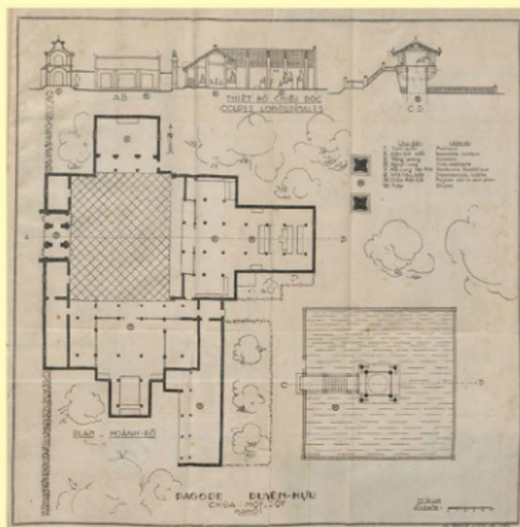
Bản vẽ Chùa Diên Hựu bao gồm Liên Hoa Đài do kiến trúc sư Lu-i Bơ-da-xi-ê (Luis Bezacier) ghi chép vào đầu thế kỷ 20 (2)
