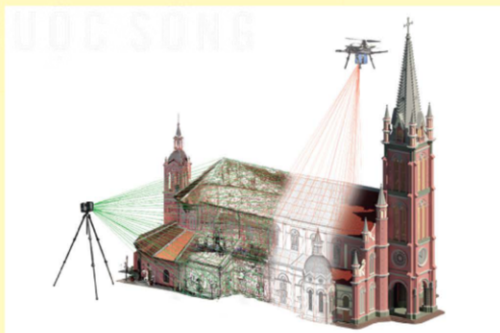
Sử dụng quét tia laser 3D trong mô hình hoá công trình kiến trúc (3)
